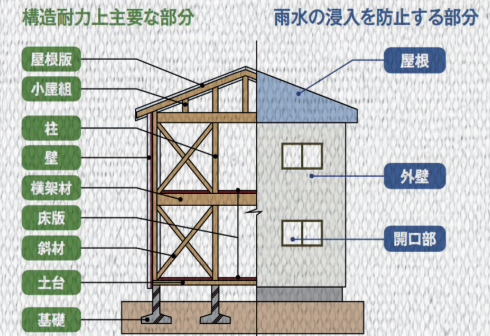
木造(軸組工法)住宅の例
